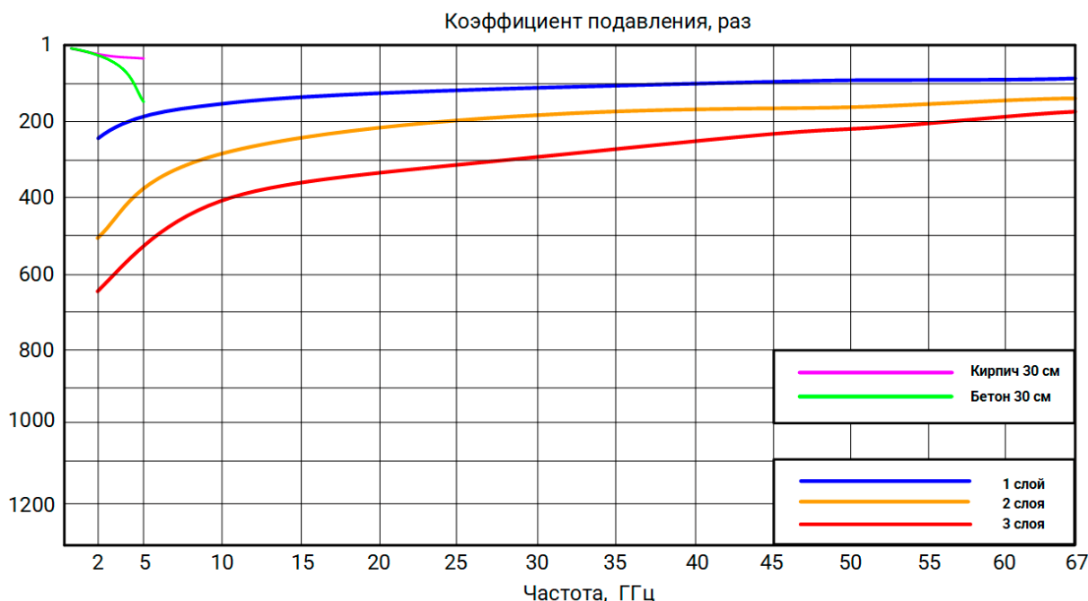
Рисунок 2 – Коэффициент подавления СВЧ-энергии волны типа Н 10 в волноводных сечениях в размах для краски РАДИОБУНКЕР 26 БАЗА
