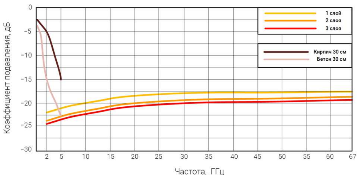
Рисунок 1 – Коэффициент подавления СВЧ-энергии волны типа Н 10 в волноводных сечениях в дБ для краски РАДИОБУНКЕР 26 БАЗА
