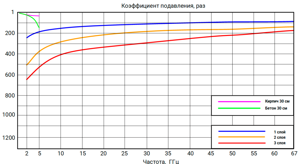
Рисунок 2 – Коэффициент подавления СВЧ-энергии волны типа H_{10} в волноводных сечениях в размах для краски РАДИОБУНКЕР 26 БАЗА
