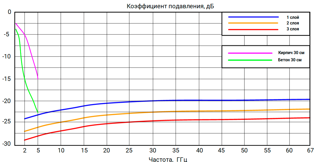
Рисунок 1 – Коэффициент подавления СВЧ-энергии волны типа H 10 в волноводных сечениях в дБ для краски РАДИОБУНКЕР 26 БАЗА
