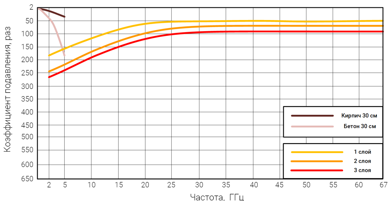
Рисунок 2 – Коэффициент подавления СВЧ-энергии волны типа Н 10 в волноводных сечениях в размах для краски РАДИОБУНКЕР 26 БАЗА
